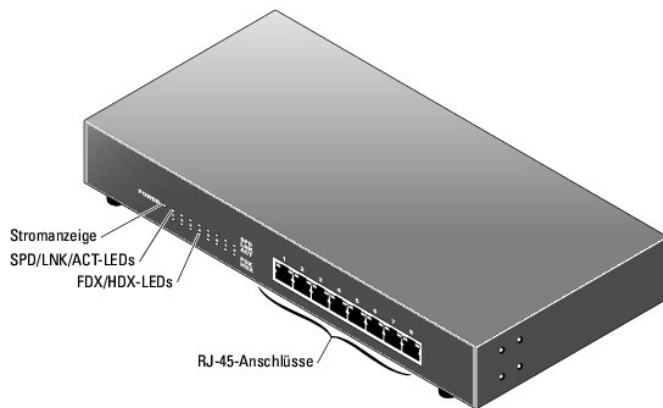
Abbildung 1-2. PowerConnect 2616
